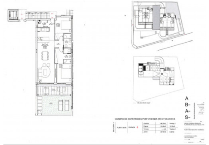
Grundriss
