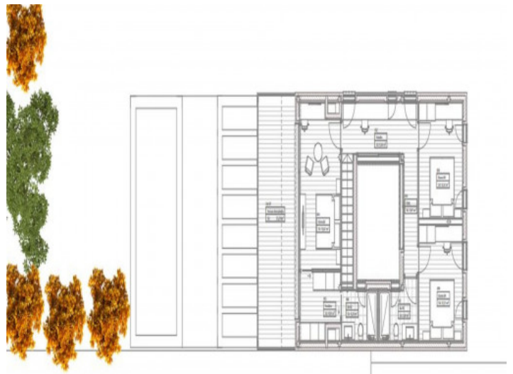
Grundriss 1. Etage
