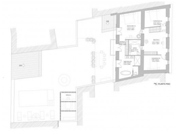
Obergeschoss
