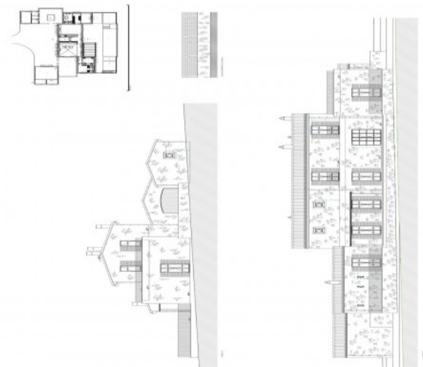
Bauplan
